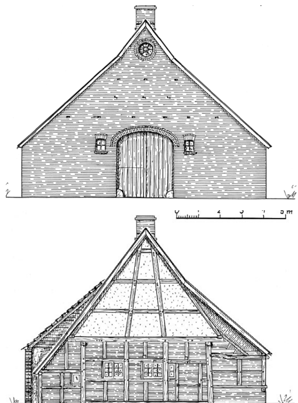
Abb. 77: Vorder- (links) und Rückgiebel (rechts) des Heuerhauses der ehemaligen Hofstelle Splanemann in Gersten (Dr. Maschmeyer)
